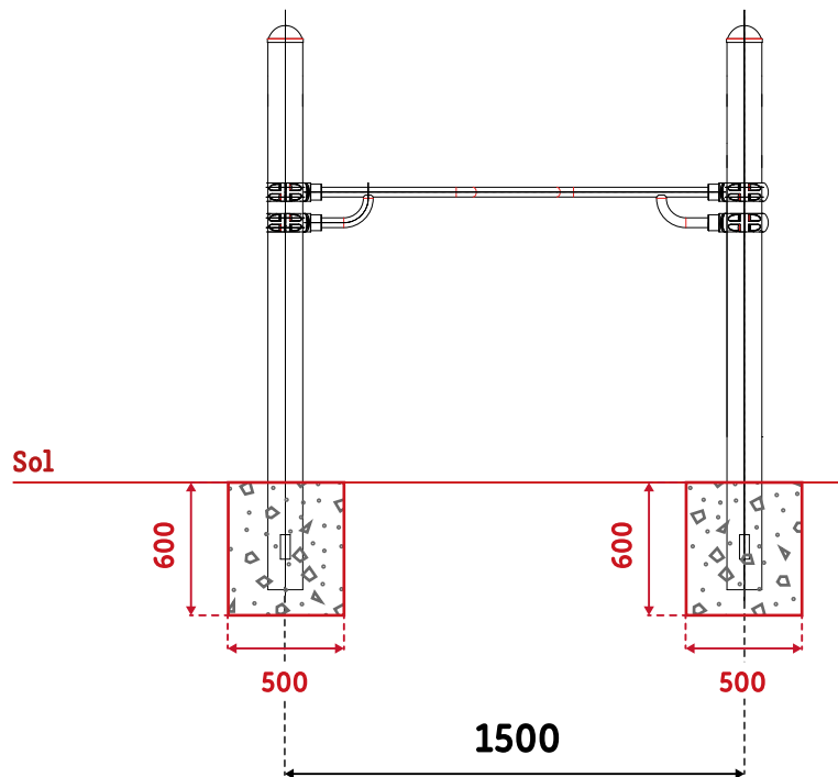
VUE LATÉRALE
