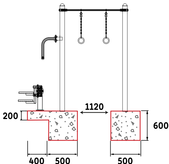
VUE LATÉRALE
