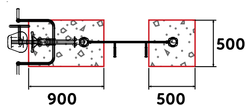
VUE DESSUS
