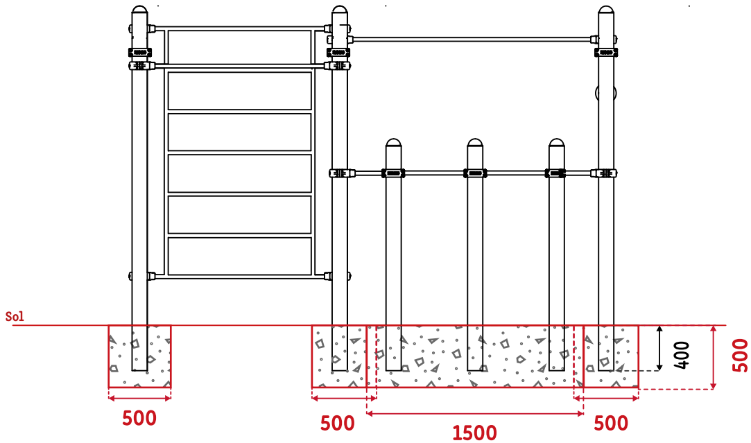
VUE LATÉRALE
