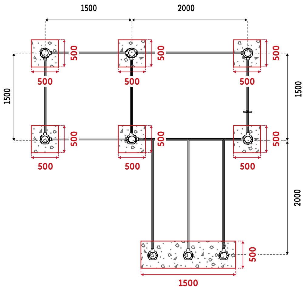
VUE DESSUS
