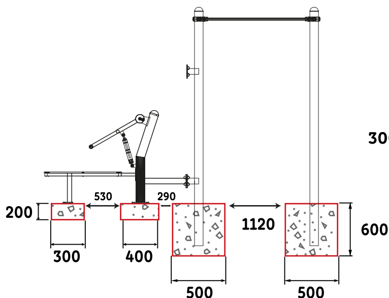
VUE LATÉRALE
